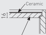
LK... lamellar finger-joint 16 mm
